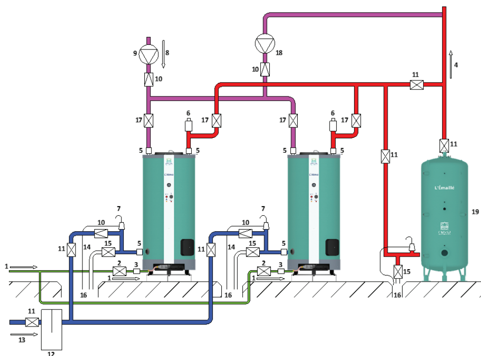
➤ Schéma de principe avec deux accumulateur et un réservoir de stockage (fig. 10)
